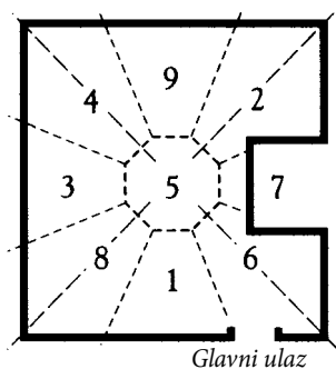
Slika br. 8: Kuća kojoj zbog proširenja neki delovi nedostaju. Ovde je polje 7, Bagve, uglavnom izvan kuće.
