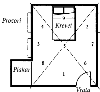
Slika br. 9: Bagva u spavaćoj sobi.
