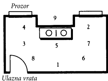
Slika br. 10: Bagva u kuhinji. Ovde nedostaju skoro cela oblast 9, i deo broja 8.
