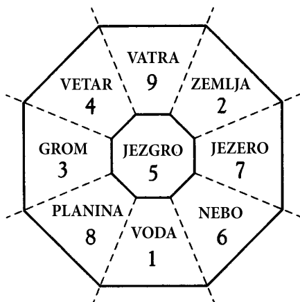
Slika 3A: Magični kvadrat se pretvara u Bagvu
