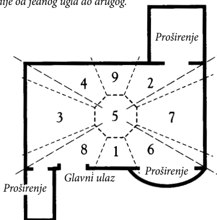
Slika br. 6: Postavljanje Bagve. Da biste našli centar sobe ili kuće nepravilnog oblika, do crtajte linije površina koje nedostaju da biste dobili imaginarni pravilni oblik, a onda povucite dve dijagonalne linije od jednog ugla do drugog.
